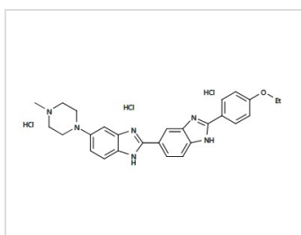
Fig. Hoechst 33342 structure formula
